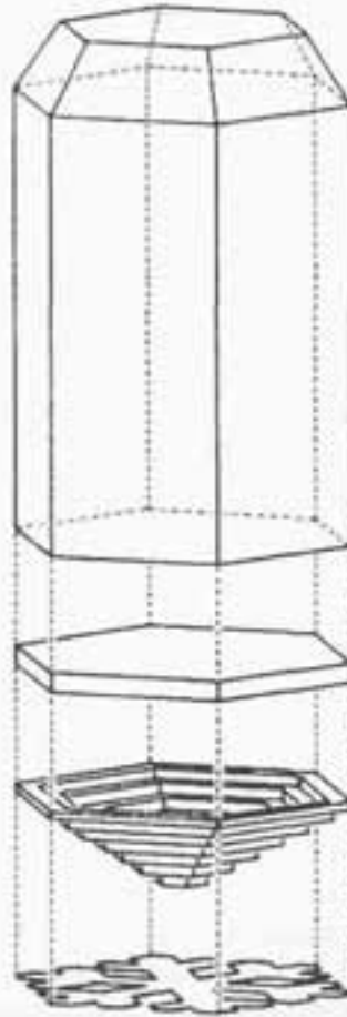
Cristales de nieve y su relación con la simetría hexagonal.
